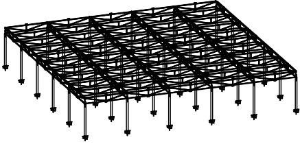
B2 Цокольний блок для монтажу на гвинтові палі або геощурупи
