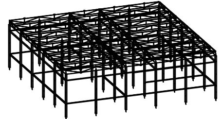
B4 Стандартний Блок поверху
